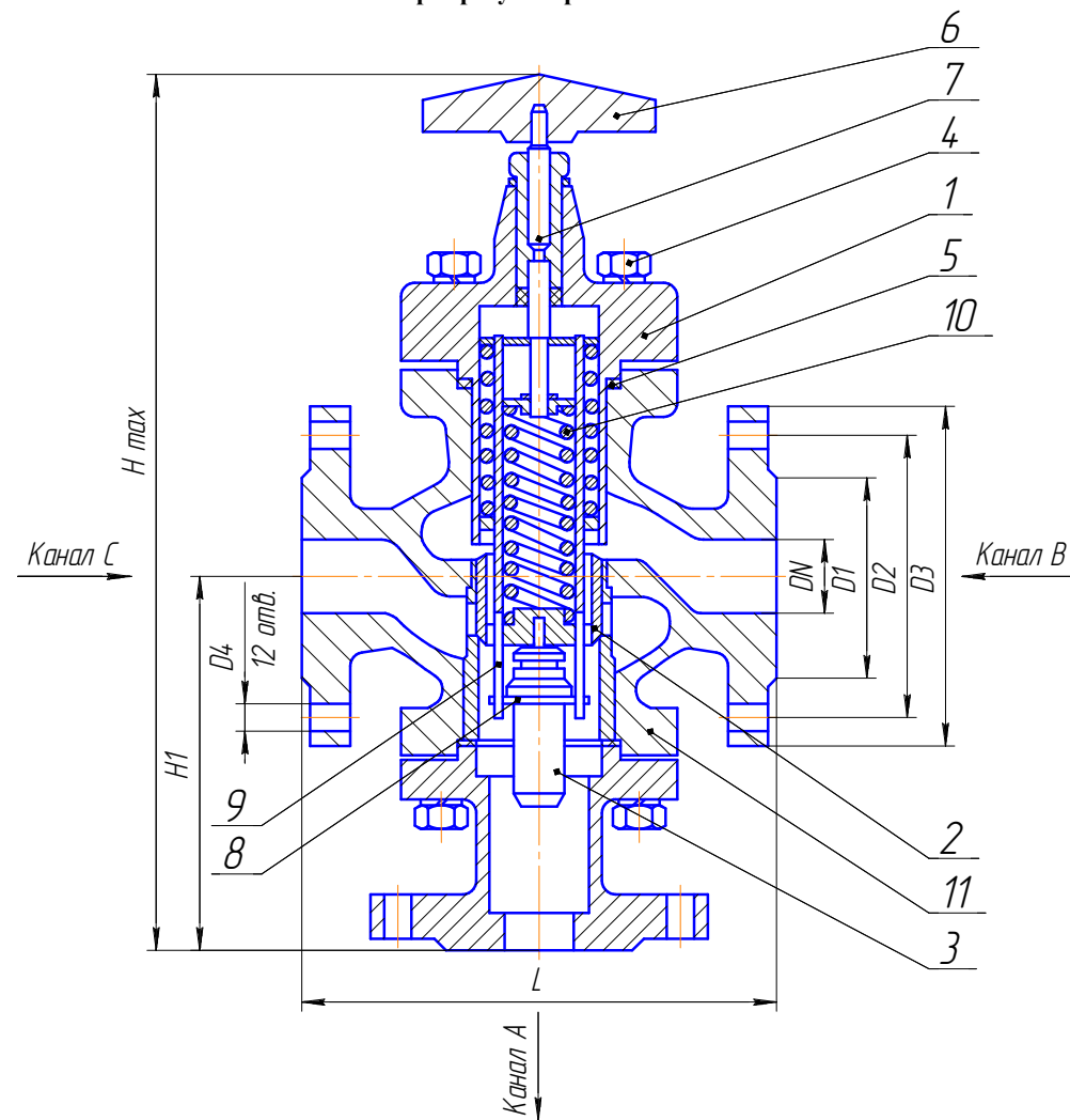
Конструкция, габаритные, установочные и присоединительные размеры терморегулятора РТ-ТС
