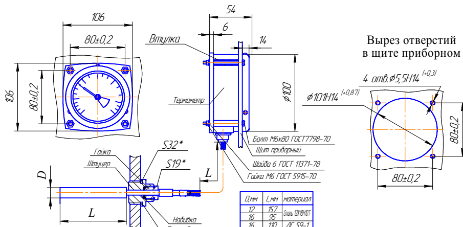
ГАБАРИТНЫЕ И ПРИСОЕДИНИТЕЛЬНЫЕ РАЗМЕРЫ ТЕРМОМЕТРА ТКП100-С
