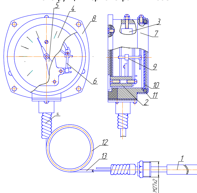
Конструкция термометра ТКП-100С
