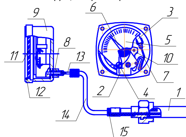
Приложение Б (справочное) Конструкция термометра ТКП-60С
