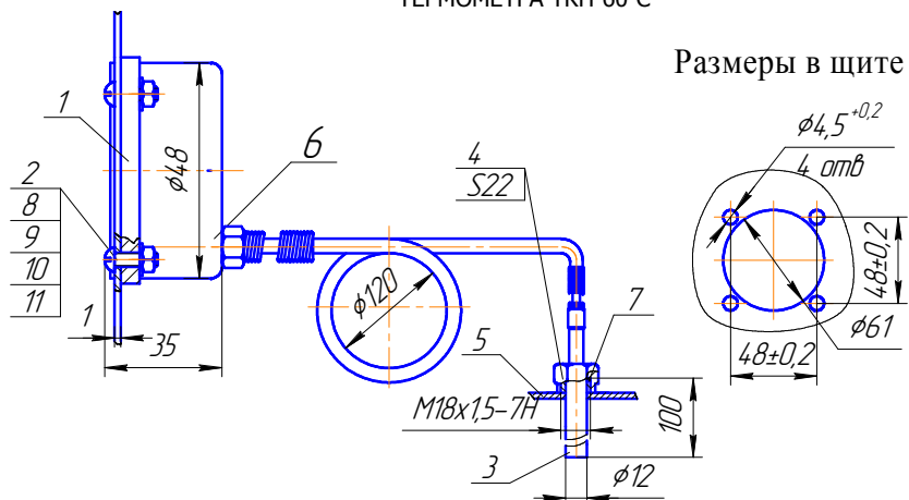
ГАБАРИТНЫЕ И ПРИСОЕДИНИТЕЛЬНЫЕ РАЗМЕРЫ ТЕРМОМЕТРА ТКП-60-С
