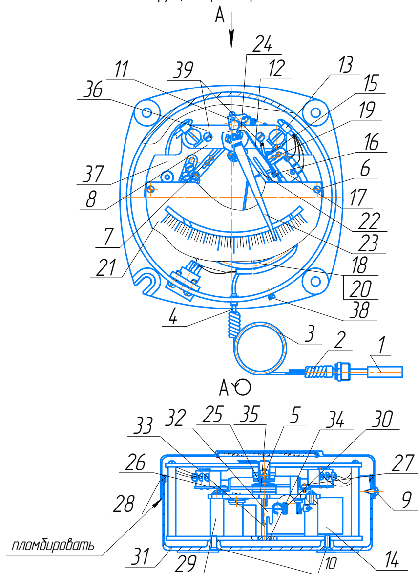
Приложение А Конструкция термометра ТКП160Сг-МЗ
