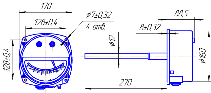
Осевые термометры ТКП-160Сг-М3
