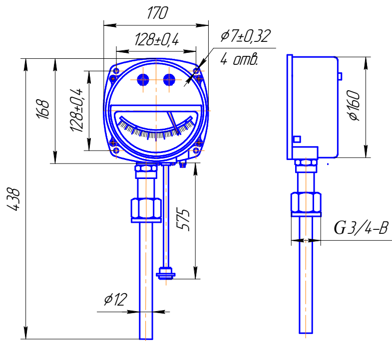
Радиальные термометры ТКП-160Сг -М3
