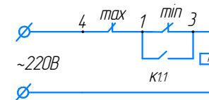
K1 – реле РП21 (или аналогичные)
