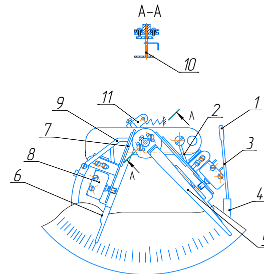
1-термобаллон; 2-поводок; 3-капилляр; 4-манометрическая пружина; 5-стрелка; 6-указатели; 7-рычаг; 8-микропереключатели; 9-тяги; 10-ось; 11-поводок.
