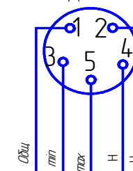
Схема внешних соединений
