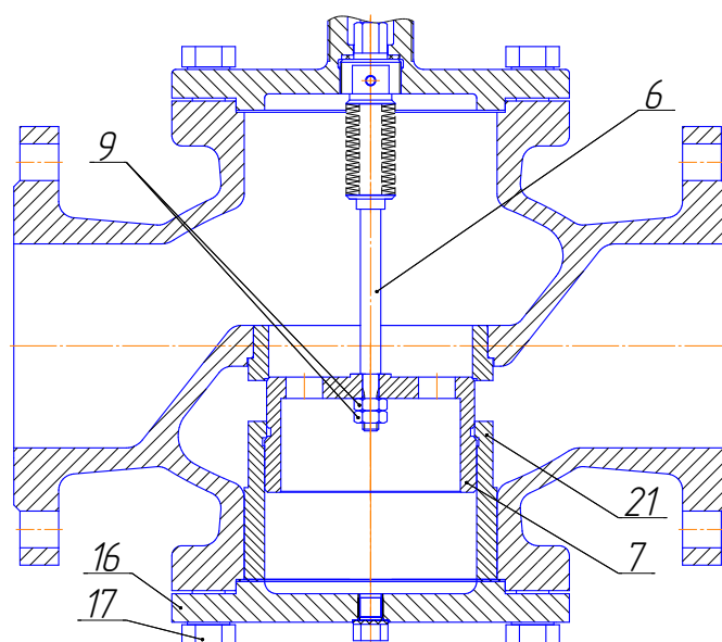
Рис. 1 Регуляторы с сильфонным уплотнением
